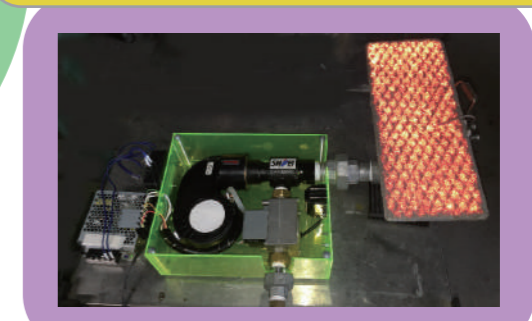
ハネウェル社プレミックスエンジン
